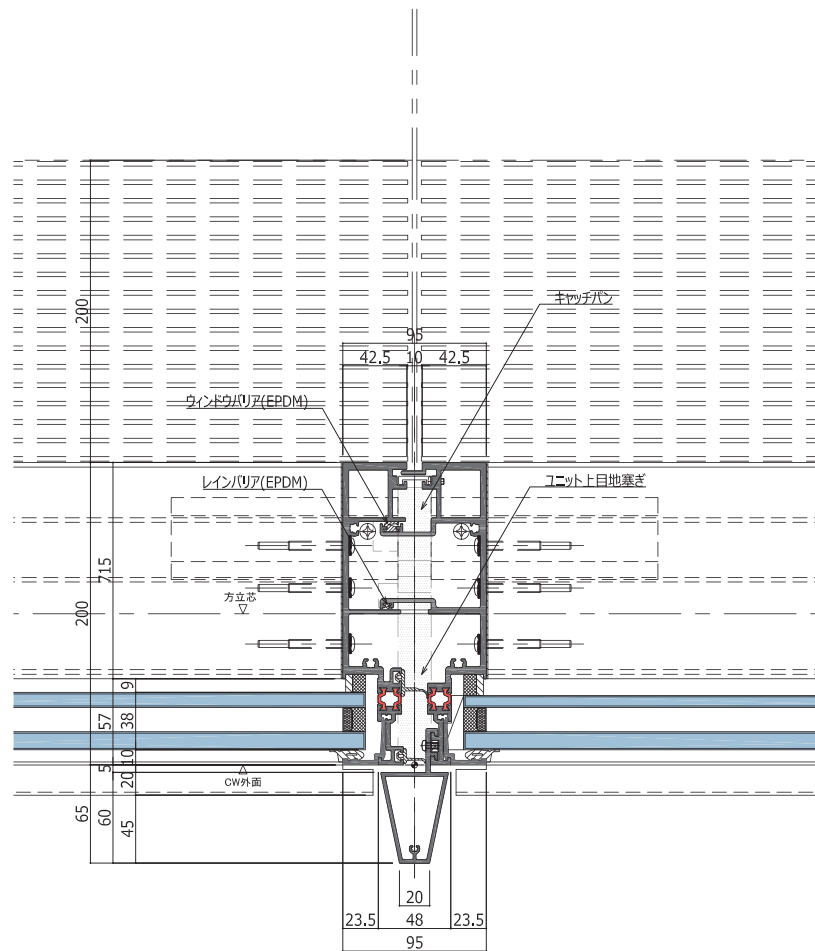
A-A 断面図 S=1/5
