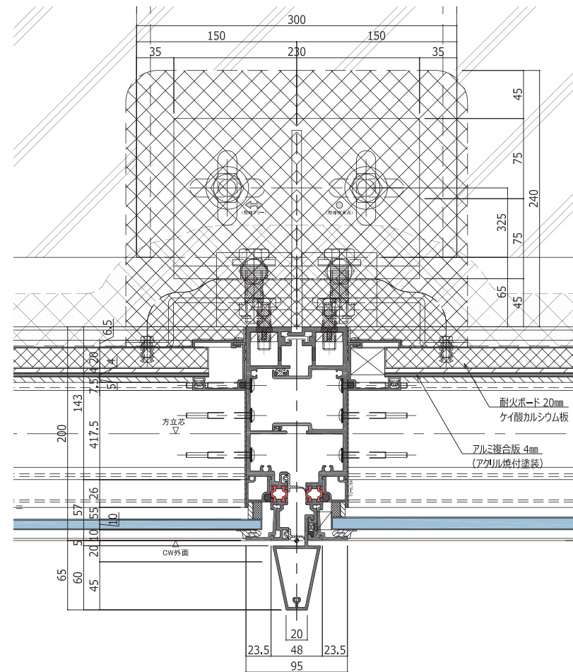
B-B 断面図 S=1/5
