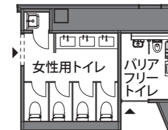
トイレ(西) 平面図
