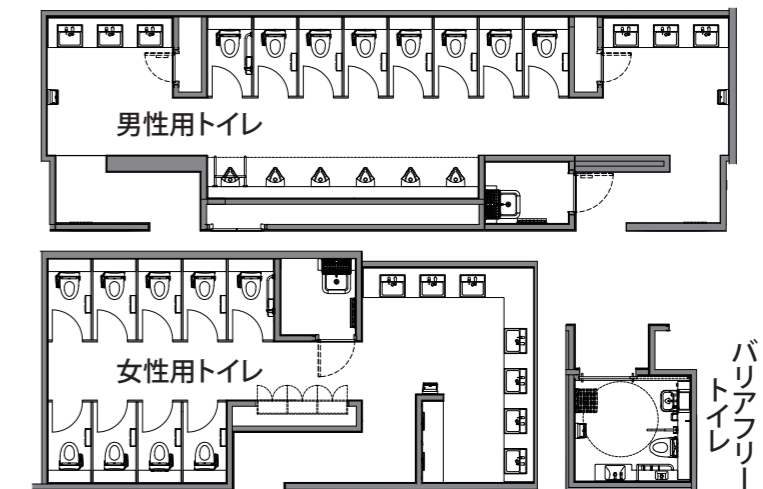
52F平面図
