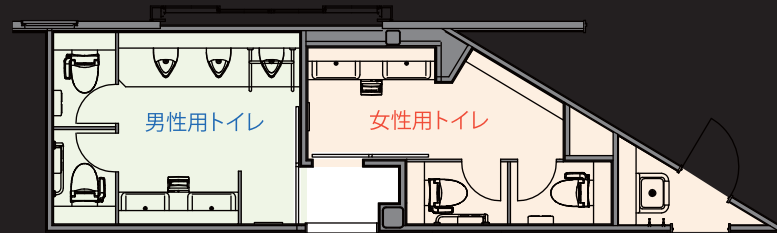
トイレ平面図
