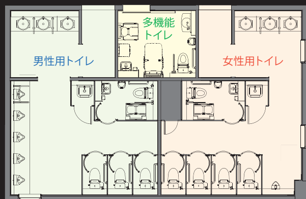
平面図
