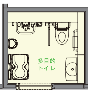
1階多目的トイレ平面図
