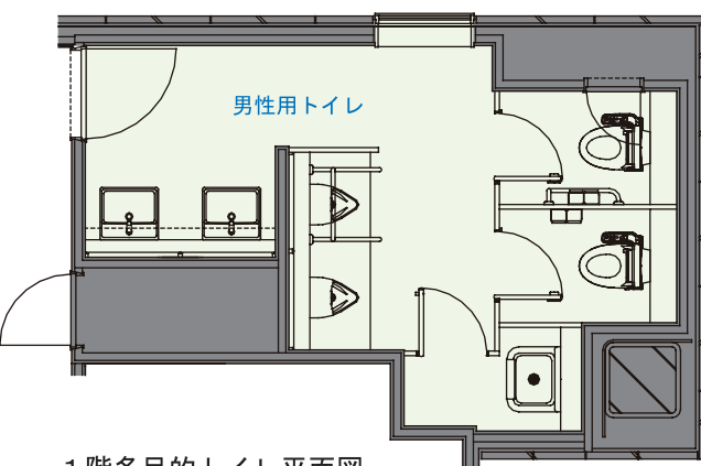
1階多目的トイレ平面図
