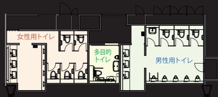
2Fトイレ 平面図
