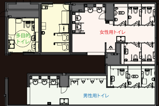
4階トイレ平面図
