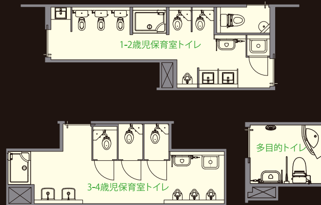
トイレ 平面図
